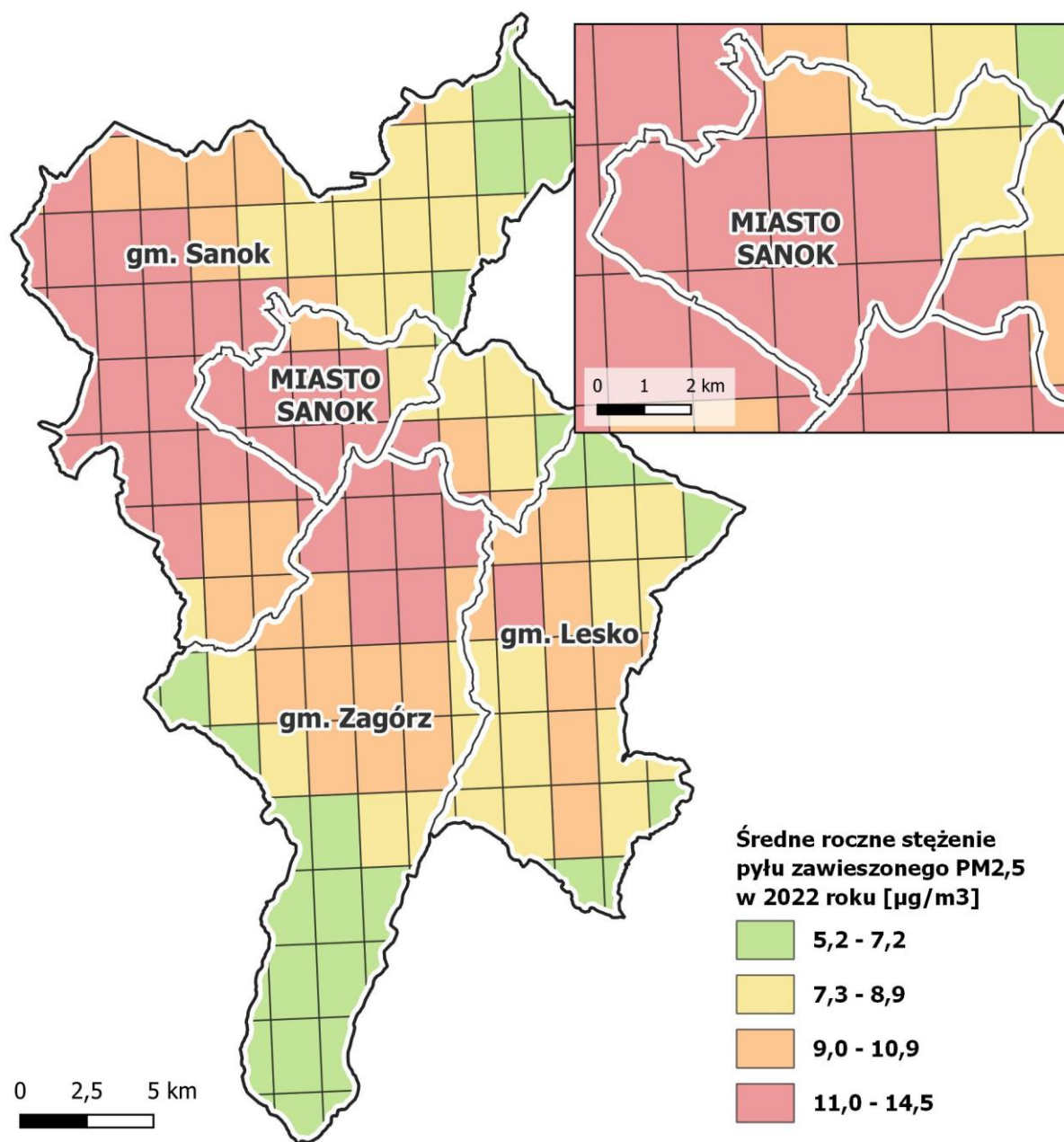
Mapa 7 Średnie roczne stężenie pyłu zawieszonego PM 2,5 w 2022 r.
